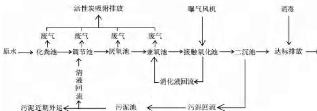
图 6 污水处理工艺流程图
